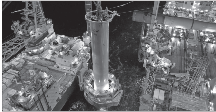
Geräuscharme Installation im Offshore-Windpark Gode Wind 3
